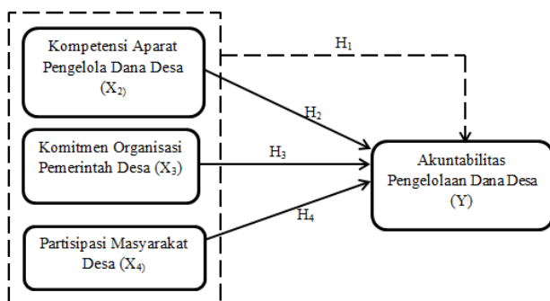
Gambar 1. Kerangka Pemikiran
